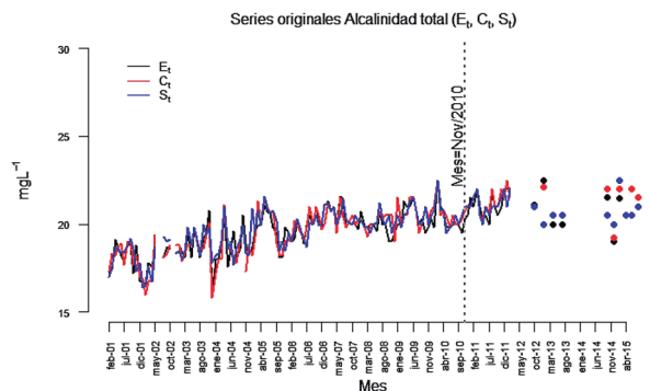
Figura 1. Comportamiento de la Alcalinidad Total (serie original) por estaciones de muestreo ( E_t , C_t y S_t ).
