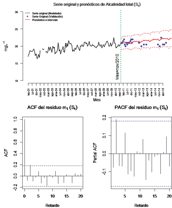
Figura 4: Serie original, valores predichos con el modelo m_1 e Intervalos de Confianza del 95%, ACF y PACF del residuo, para Alcalinidad Total en la Salida.
