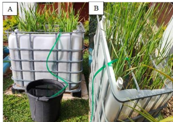
Figura 2. (A) Vista general del sistema alimentado semanalmente (B) Adaptación y crecimiento de macrófitas, sin signos de fitotoxicidad en tres meses de operación del sistema.
