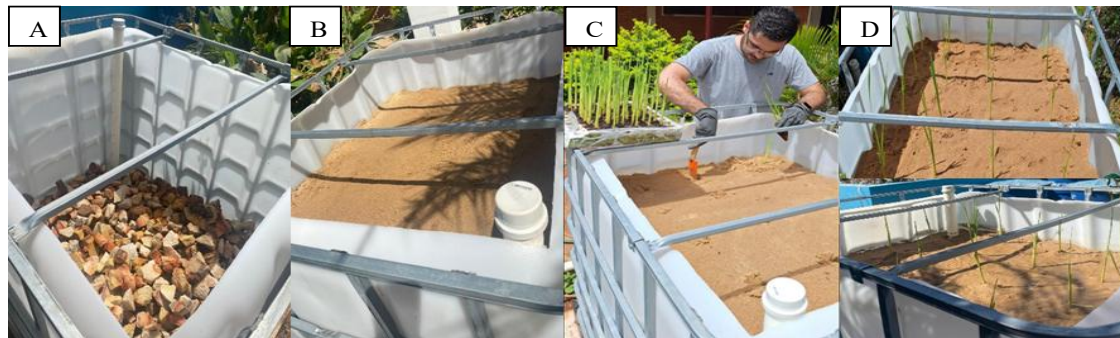
Figura 1. (A) Acondicionamiento con gravas capa inferior e intermedia, (B) Capa superficial arena gruesa (C) siembra de macrófitas en el humedal (D) plantines sembrados.
