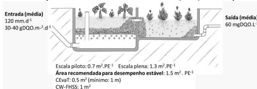
Figura 1. Vista da seção transversal do sistema de EvaTAC e principais condições estudadas.
